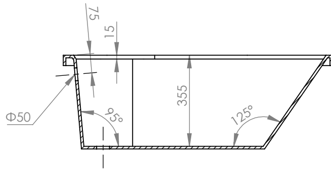
SECTION A-A SCALE 1 : 15
